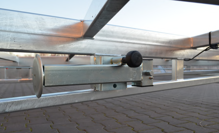
Stützbeine für Anhänger (4x 1300 kg)
