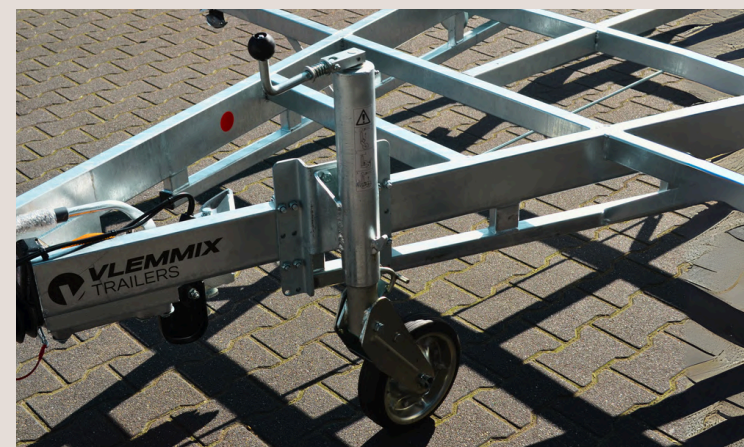
Stützrad 800 kg inkl. Stützradhalter
