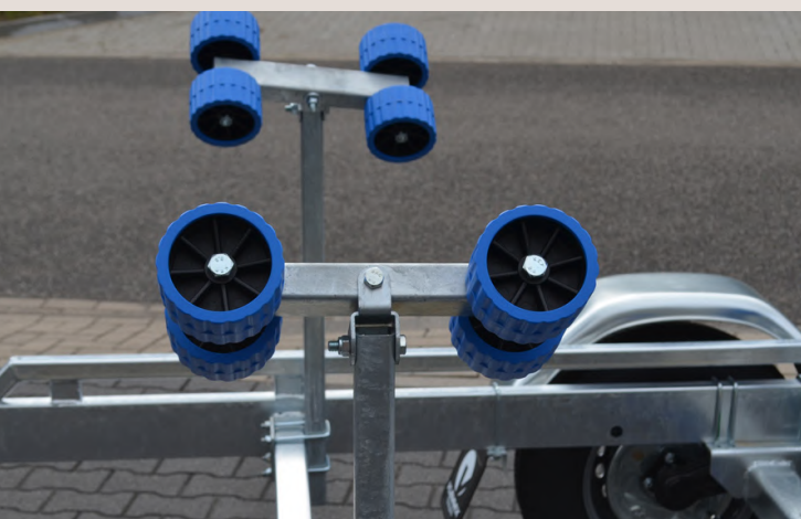
Double keel rollers
