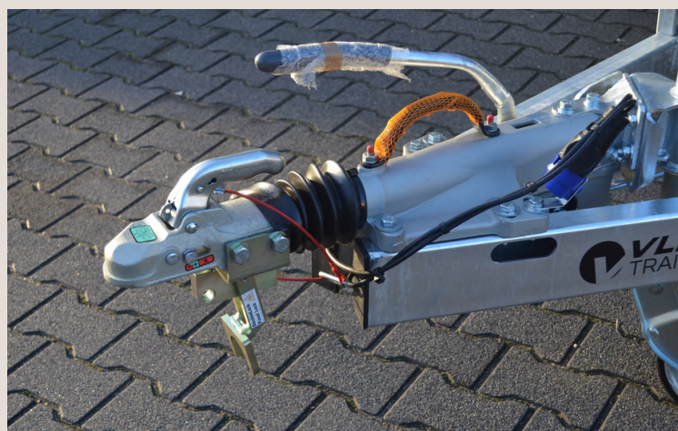
SCM-geprüftes Schloss
