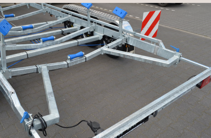
V-Konstruktion
