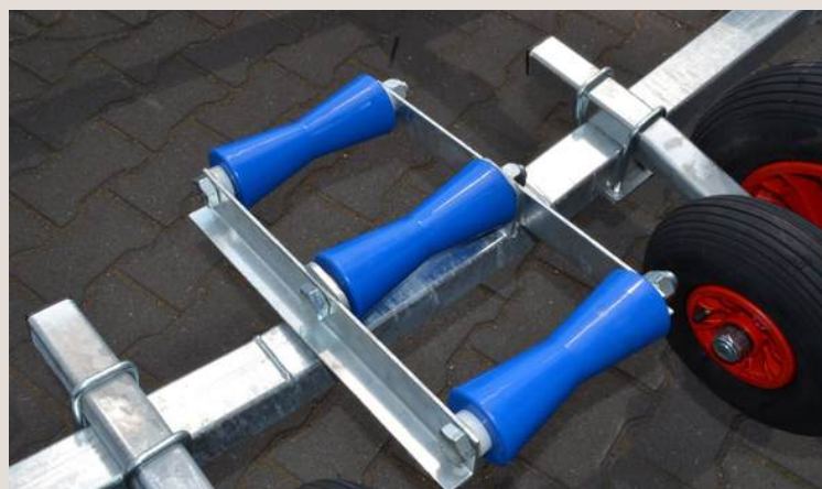
Kielrol kantelsysteem
